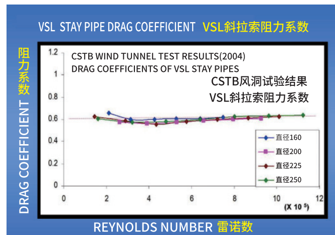
风洞实验
