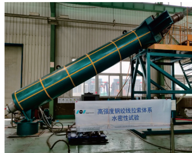
■ 水密性实验
