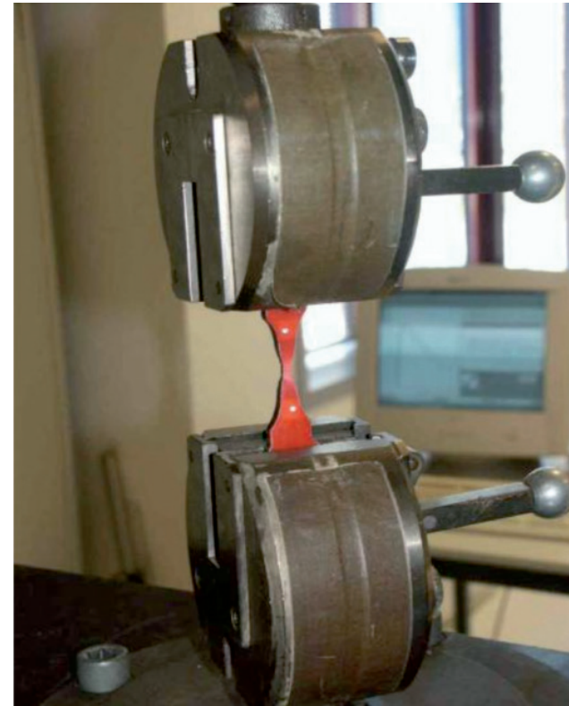
■ 加速老化实验后对HDPE外套管进行张拉实验
