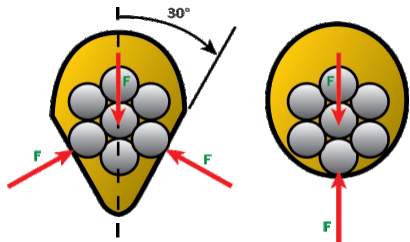
SSI鞍座截面，“V”型钢绞线导向孔与圆形导向孔比较
